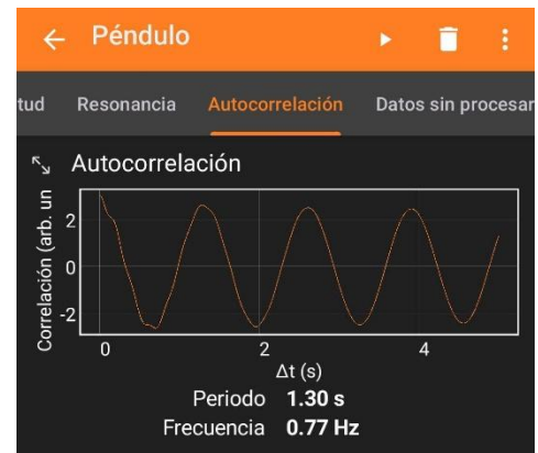
Ilustración 3: Gráfica de PHYPHOX de autocorrelación
