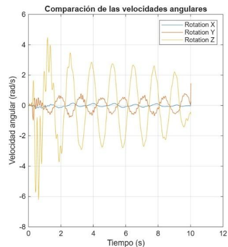
Ilustración 10: Gráfica de MATLAB, comparación de velocidad
