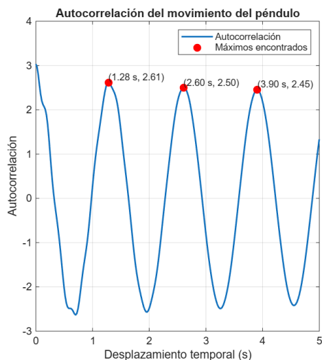
Ilustración 15: Gráfica PYTHON, autocorrelación del movimiento
