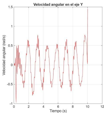
Ilustración 6: Gráfica de MATLAB velocidad angular eje y
