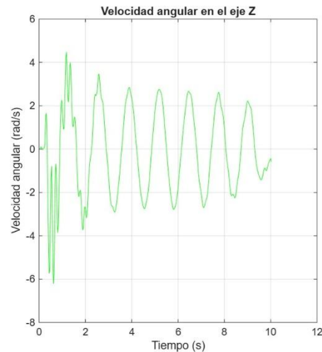
Ilustración 7: Gráfica de MATLAB velocidad angular eje z
