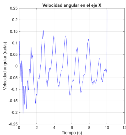
Ilustración 12: Gráfica PYTHON velocidad angular eje X
