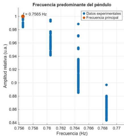
Ilustración 8: Gráfica de MATLAB frecuencia predominante
