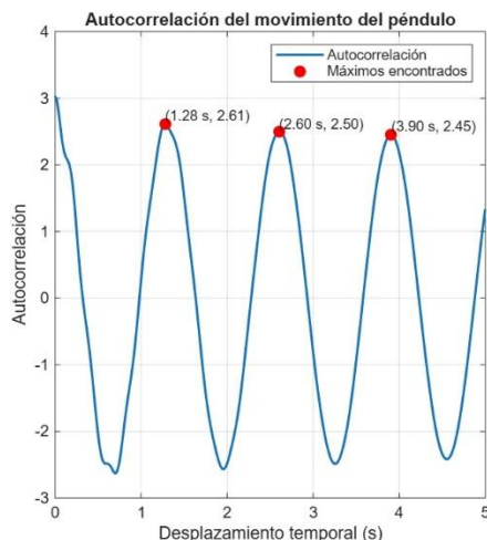
Ilustración 9: Gráfica de MATLAB de Autocorrelación
