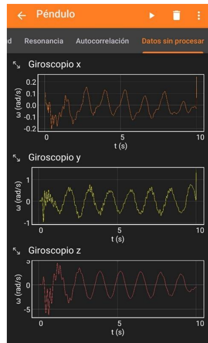
Ilustración 2: Grafica de PHYPHOX en los eje X,Y,Z
